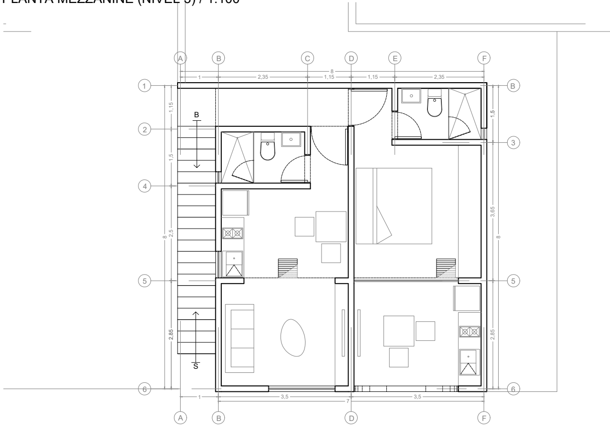
PLANTA ALTA ARQUITECTÓNICA / 1:100
