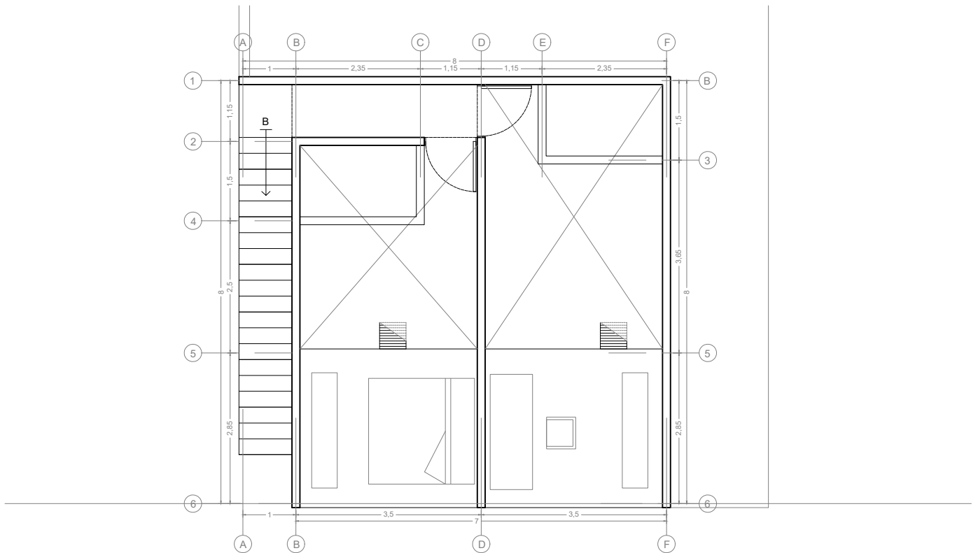
PLANTA MEZZANINE (NIVEL 3) / 1:100
